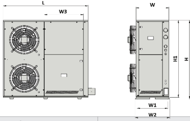
DIŞ ÜNİTE / OUTDOOR UNIT = 276 kg
